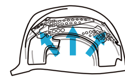
エアロメッシュ®が伸びて吸収
